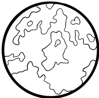
Moon
