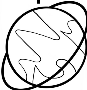
Uranus
